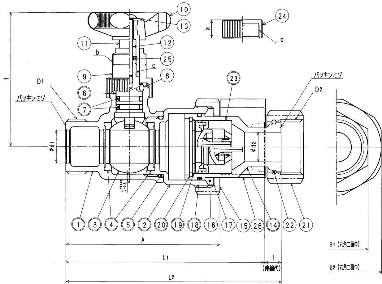
寸法表
